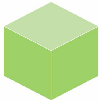
ඝණකය
