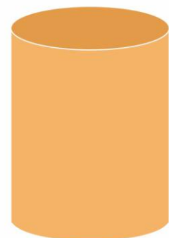
සිලින්ඩරය
